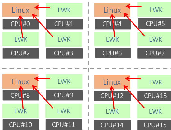
Figure 1.4: ihk_os_set_ikc_map() の例
