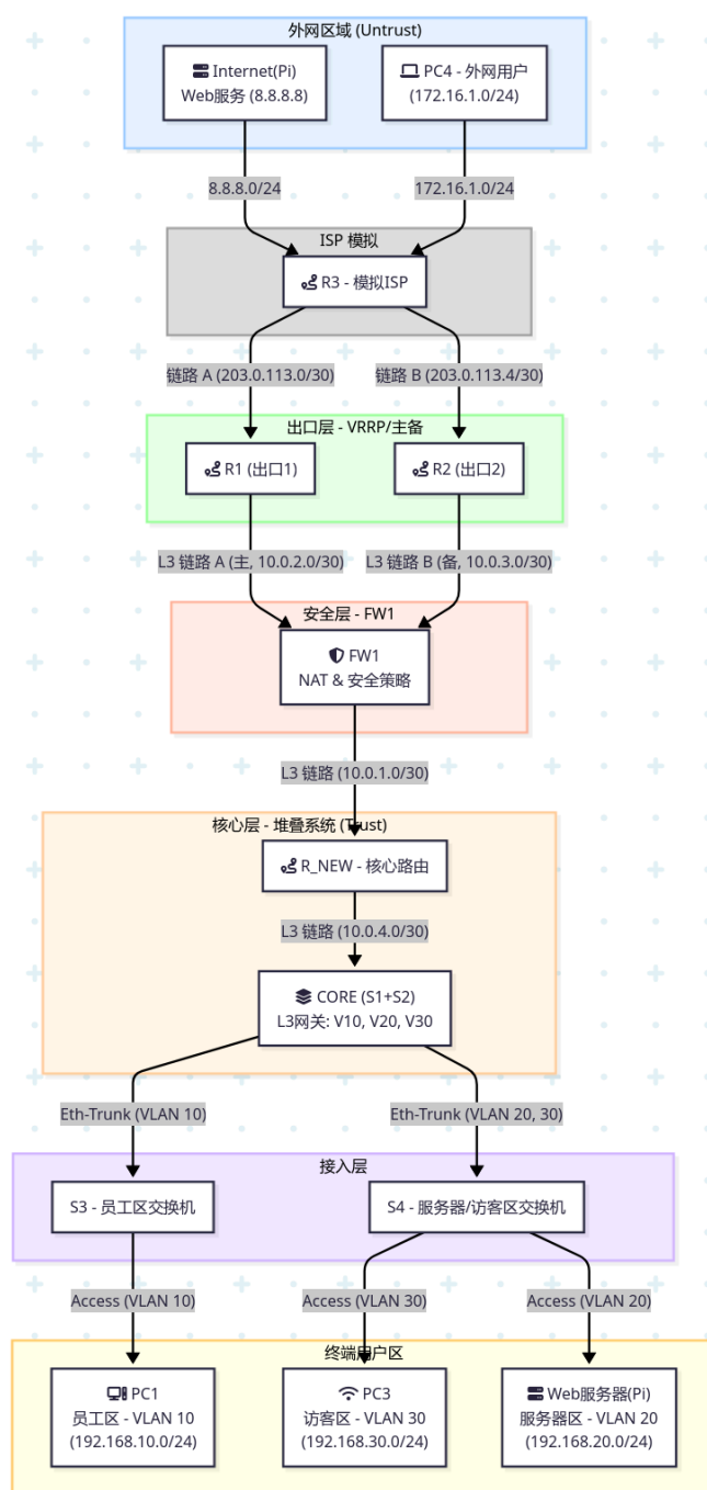
Figure 2: 实验示意图
