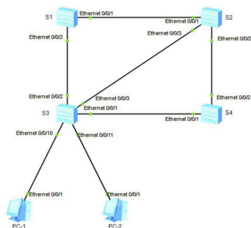
图 6 实验拓扑图
