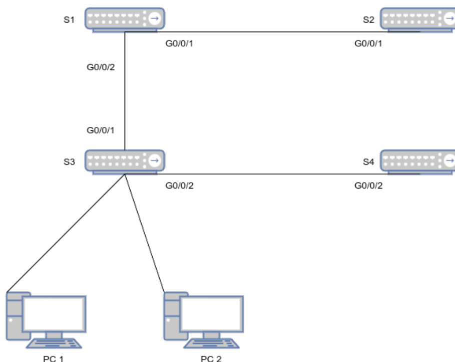
图 21 查看阻断后的拓扑
