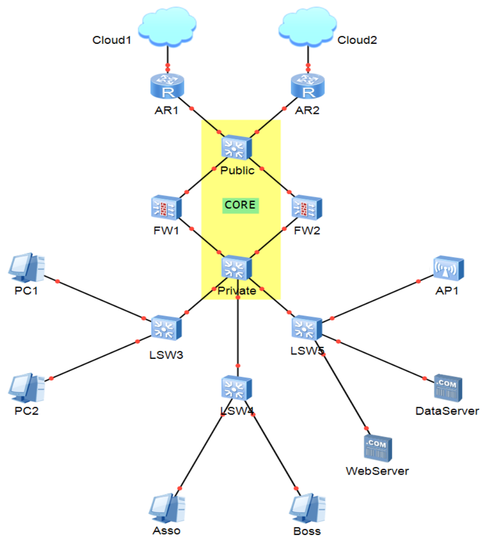
Figure 9: 逻辑拓扑图（完整）
