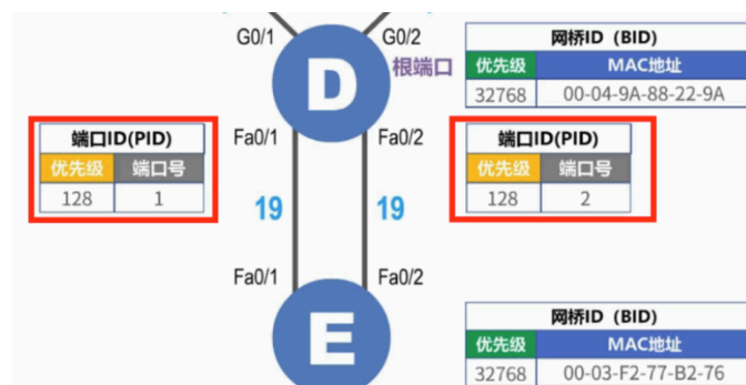
Figure 4: 对端 PID 最小
